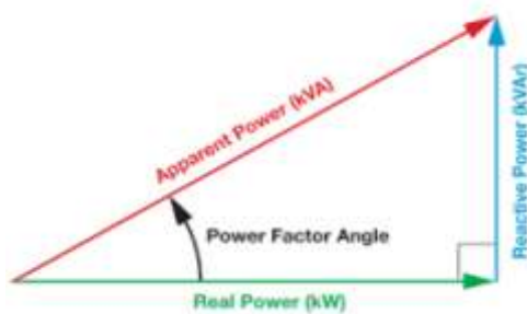
Fig A: Power Triangle
