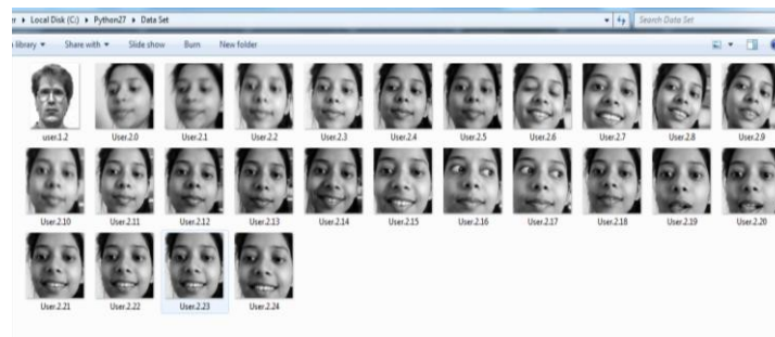
Fig.5.1. Prepare Dataset
