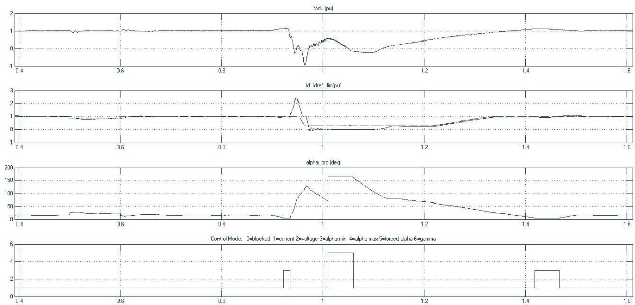
Figure4: Rectifier DC quantities
