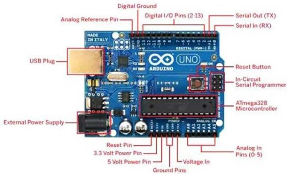
Fig 4.2 Arduino UNO
