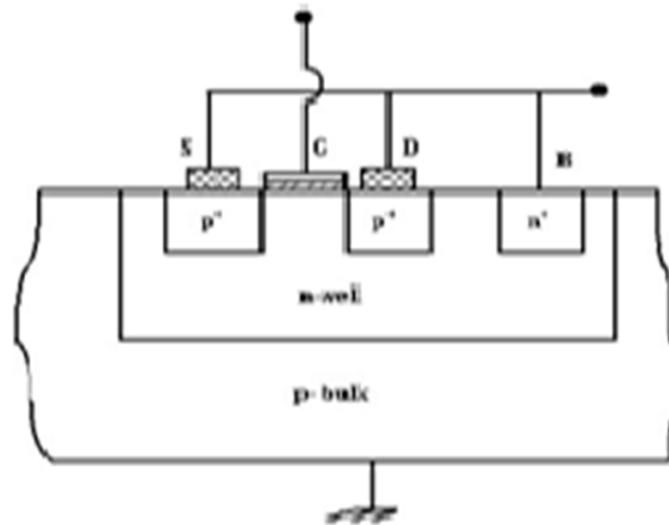
Fig.3. MOS Capacitor
