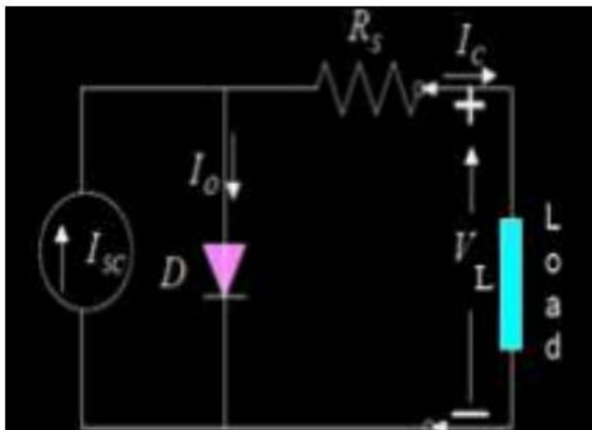
Fig: 1. PV cell
